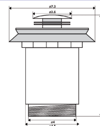
VÁLVULA CLIC CLAC LAVATÓRIO/BIDÉ SEM FURO
