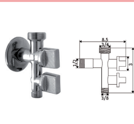
TORNEIRA CORTE DUPLA TML
