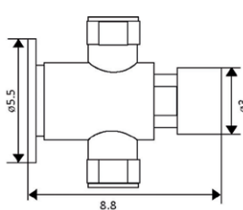
TEMPORIZADOR PARA PASSADOR EXTERIOR IDRAL
