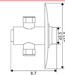
TEMPORIZADOR PARA TORNEIRA TEMP. IDRAL
