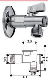
TORNEIRA CORTE COM FILTRO LONGO C/ MANÍPULO METAL
