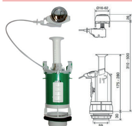
VÁLVULA DESCARGA OLI DUPLA COM CABOS
