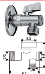
TORNEIRA CORTE COM FILTRO PEQUENA TML
