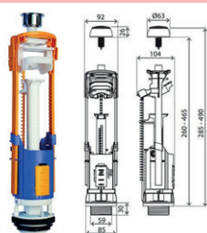
VÁLVULA DESCARGA OLI ATLAS DD
